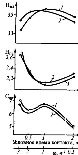
Рис. 3.15. Влияние объемной скорости подачи сырья \omega на характеристики ароматического ядра "средней молекулы" гидрогенизатов [в % (мас.)] при температурах гидроочистки 360°C (1) и 380°C (2)
