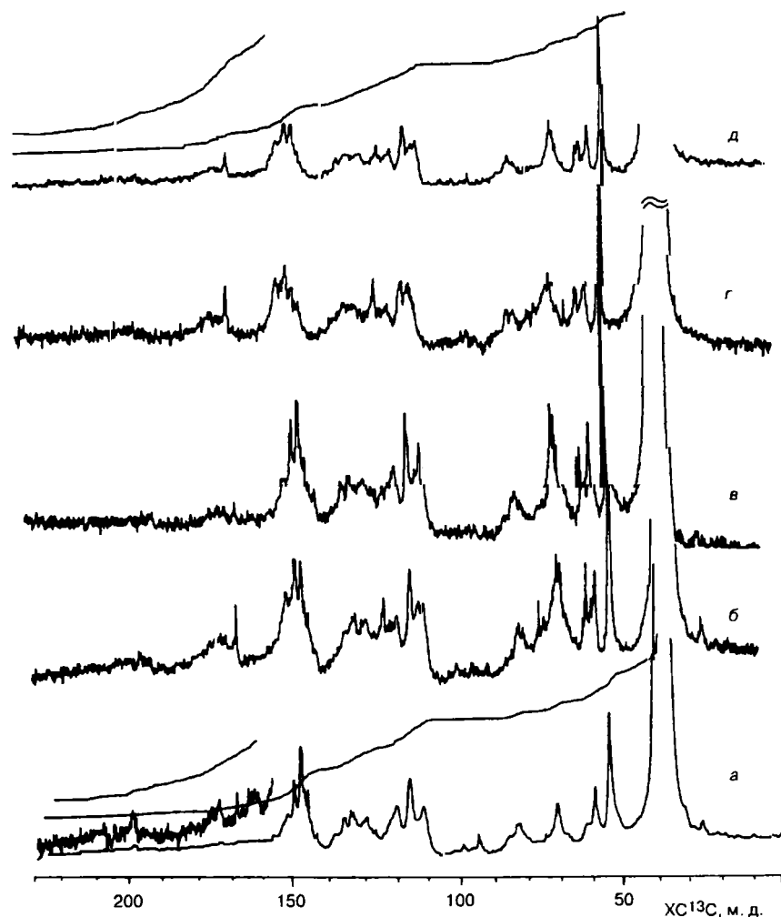
Рис. 2.22. Спектры ЯМР ^{13}\text{C} лигнинов лиственницы, выделенных из здоровой (а) и разрушенной грибом Ph. sanguinea (б–д) древесины
