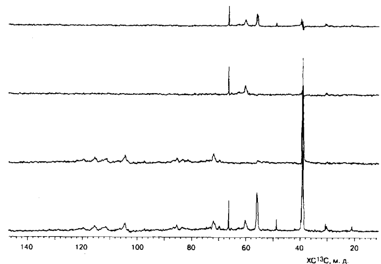
Рис. 2.6. Общий спектр ЯМР ^{13}\text{C} (а) и подспектры \text{CH} (б), \text{CH}_2 (в), \text{CH}_3 (г) ДЗС хлопчатника, полученные по методике DEPT
