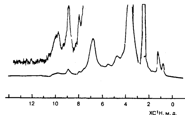
Рис. 2.3. Спектр ЯМР 1 H ДЗС в растворе ГМФА-D 18
