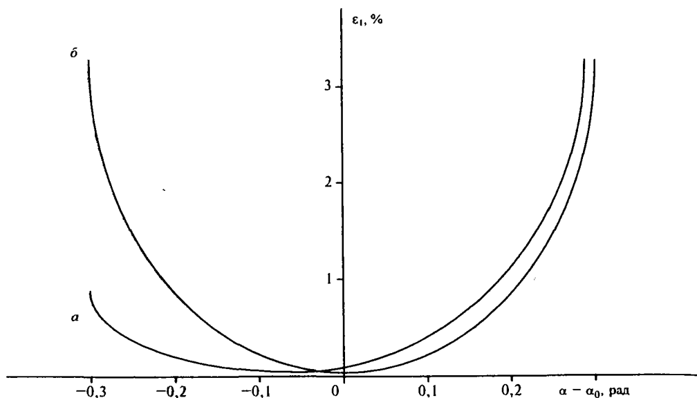
Рис. 1.17. Зависимость погрешности \varepsilon_1 от дефекта опрокидывающего импульса при \beta = 0 (а) и \beta = 0,464 рад (б)
