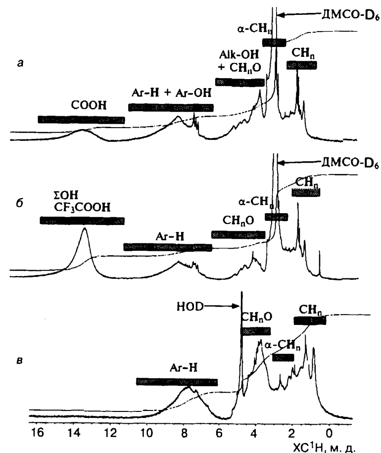
Рис. 4.5. Спектры ЯМР ^1\text{H} препарата в \text{DMSO-D}_6 (а), в \text{DMSO-D}_6 с добавкой \text{CF}_3\text{COOH} (б) и в 0,1 M растворе \text{NaOD} в \text{D}_2\text{O} (в) [484]
