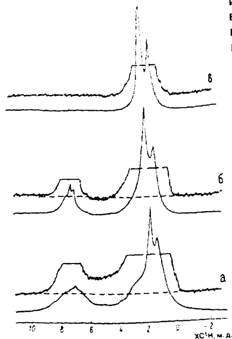
Рис. 3.13. Спектры ЯМР ^1\text{H} асфальтенов в условиях импульсного эксперимента спинового эха:
