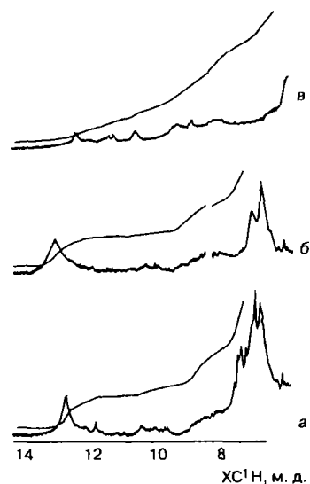
Рис. 2.1. Область спектров ЯМР ^1\text{H} групп \text{OH}_{\text{ар}} , \text{COH} , \text{COOH} препаратов ДЛМ (а), ДЛХ (б), ДЛП (в) в растворе ГМФА- \text{D}_{18}
