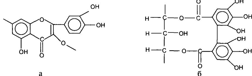
Рис. 2.19. Фрагменты структур танинов
