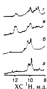
Рис. 1.10. Область спектров ЯМР ^1\text{H} гидроксильных групп ЛМРЕ (а), ЛМРЛ (б), ЛМРО (в), ДЛО (г) в растворителе ГМФА- \text{D}_{18}
