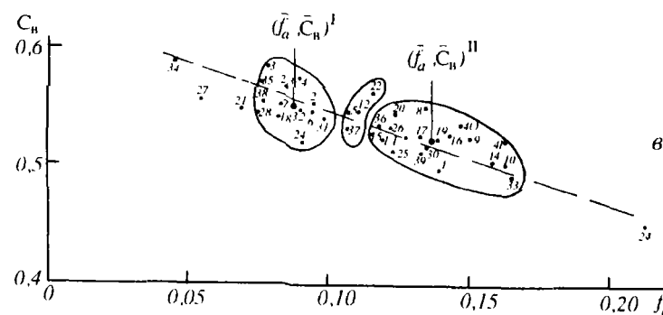
Рис. 3.1. Распределение нефтей юга Сибирской платформы (1—41) в факторном пространстве после факторизации данных ЯМР ^{13}\text{C} (а), ЯМР ^1\text{H} (б) и зависимость для них содержания вторичных алифатических углеродных атомов от ароматичности (в)
