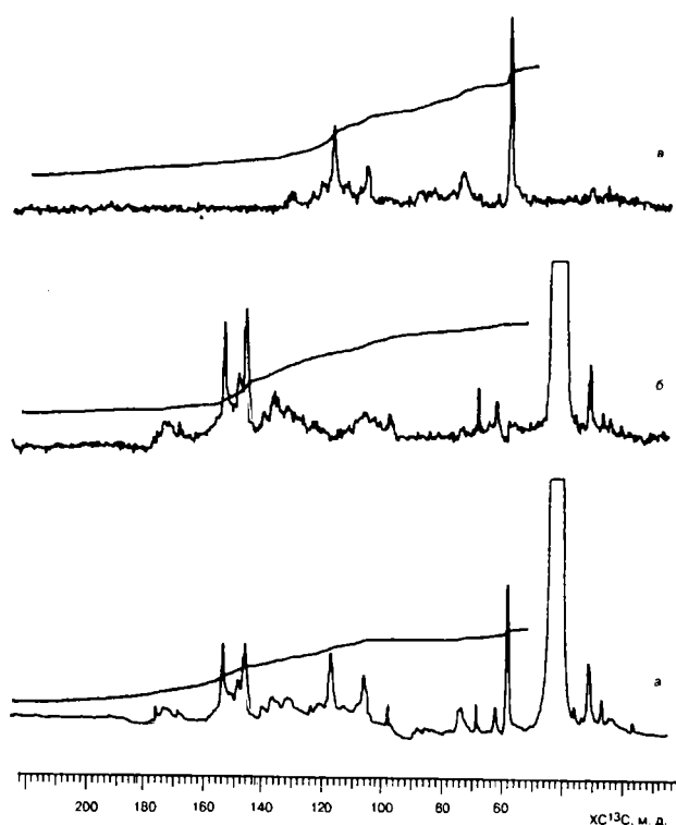
Рис. 2.15. Спектр ЯМР ^{13}\text{C} (а) и подспектры вторичных и четвертичных (б), первичных и третичных (в) атомов углерода ДПС хлопчатника в растворе \text{DMCO-D}_6
