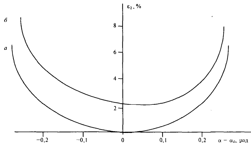
Рис. 1.18. Зависимость погрешности \varepsilon_2 от дефекта инвертирующего импульса при \beta = 0 (а) и \beta = 0,149 рад (б)
