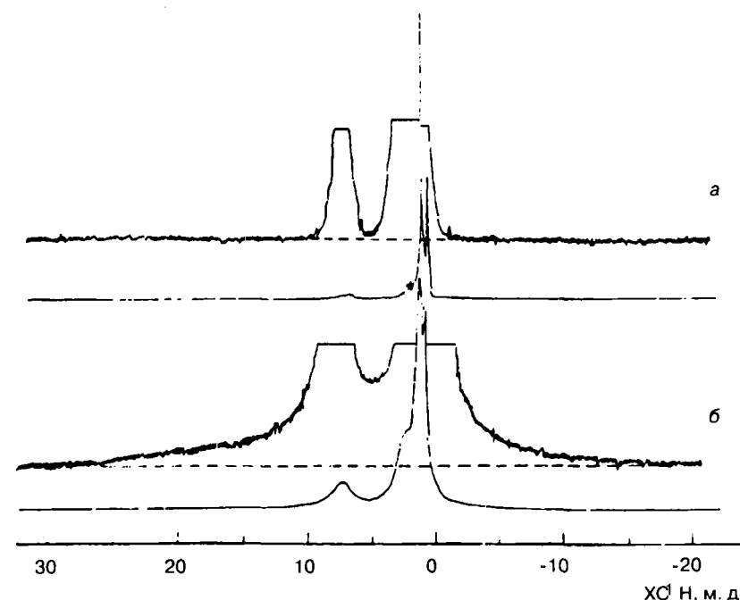
Рис. 3.8 Границы распределения спектральной плотности протонов в спектрах ЯМР ^1\text{H} мальтенов (а), асфальтенов (б) арланского гудрона. Растворитель \text{CCl}_4 , концентрация 7% (мас.), ширина развертки 50 м.д.
