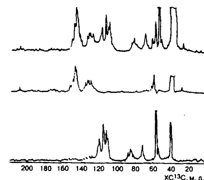
Рис. 2.29. Спектр ЯМР ^{13}\text{C} лигнина 1 (а); подспектры вторичных и четвертичных (б), первичных и третичных (в) атомов углерода
