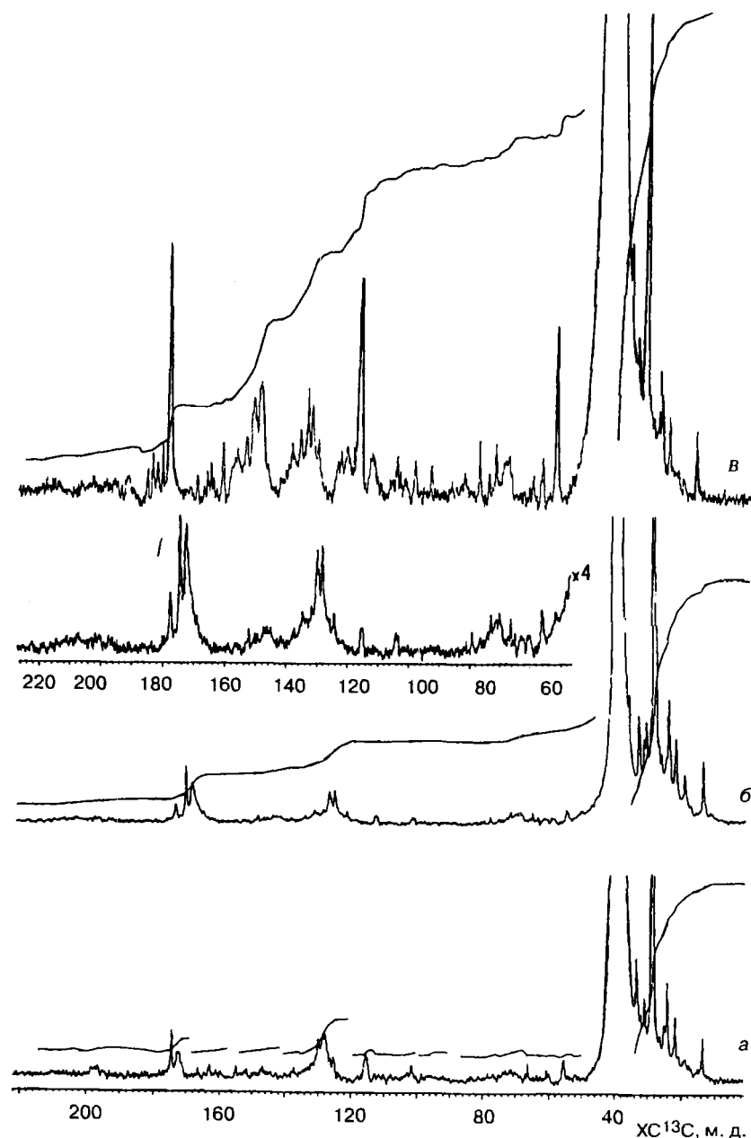
Рис. 2.2. Спектры ЯМР ^{13}\text{C} препаратов ДЛМ (а), ДЛХ (б), ДЛП (в)
