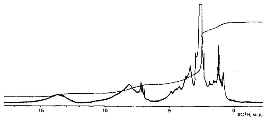
Рис. 4.4. Спектр ЯМР ^1\text{H} ГК почв, растворитель — \text{DMSO-D}_6 [483]
