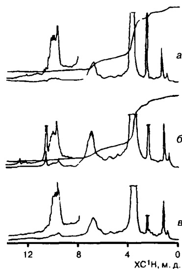
Рис. 2.27. Спектры ЯМР ^1\text{H} диоксанлигнина ели (а); ДЛЕ, обработанного \text{H}_2\text{O}_2 (б) и ДЛЕ, обработанного \text{NaBH}_4 (в)
