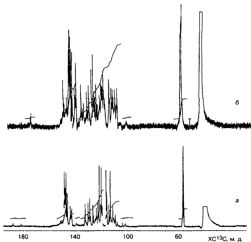
Рис. 2.33. Спектры ЯМР ^{13}\text{C} полимеров 1 (а) и 2 (б)
