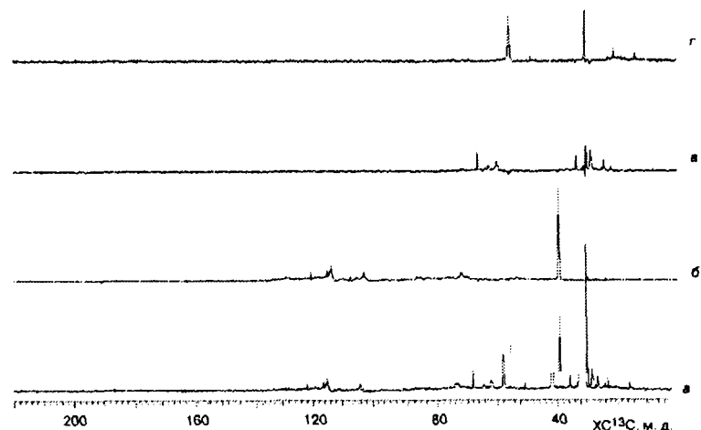
Рис. 2.18. Общий спектр ЯМР ^{13}\text{C} (а) и подспектры \text{CH} (б), \text{CH}_2 (в), \text{CH}_3 (г) ДОС хлопчатника, полученные по методике DEPT
