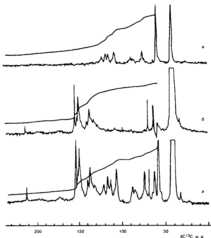
Рис. 2.14. Спектр ЯМР ^{13}\text{C} (а) и подспектры вторичных и четвертичных (б), первичных и третичных (в) атомов углерода ДЗС хлопчатника в растворе \text{DMCO-D}_6
