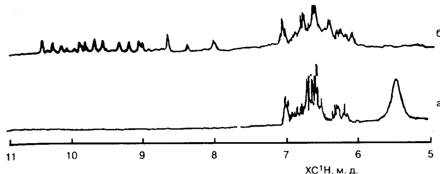
Рис. 1.7. Область спектра ЯМР ^1\text{H} атомов водорода ароматических колец и фенольных OH-групп смеси фенолов в растворителе \text{CDCl}_3 (а) и ГМФА- \text{D}_{18} (б)
