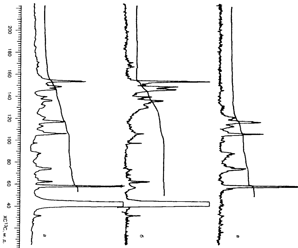
Рис. 2.16. Спектр ЯМР ^{13}\text{C} (а) и подспектры вторичных и четвертичных (б), первичных и третичных (в) атомов углерода ДПС хлопчатника в растворе \text{DMCO-D}_6
