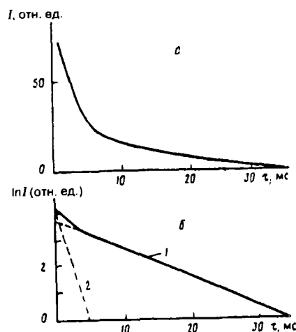
Рис. 3.9. Зависимость интегральной интенсивности I сигнала протонов нефтяных асфальтенов от времени задержки \tau в последовательности ( 90^\circ - \tau - 180^\circ ) (а) и ее графическая обработка методом касательных (б). Прямая 1 определяется соотношением \ln I_2 = \ln I_{02} - \tau/T_{22} , при больших \tau I_2 = I ; прямая 2 — соотношением \ln(I - I_2) = \ln I_{01} - \tau/T_{21}
